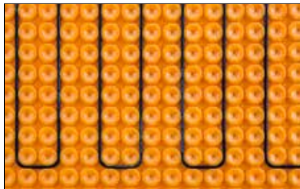
Verlegeabstand 6 cm - um jede 2. Noppe
